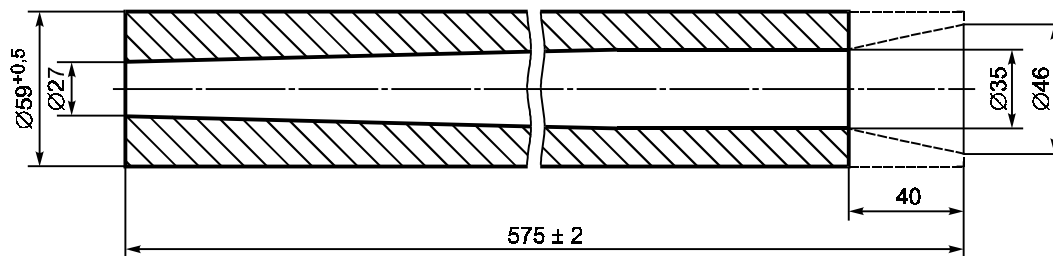
Рисунок Е.7 — Полиуретановая трубка из материала А
